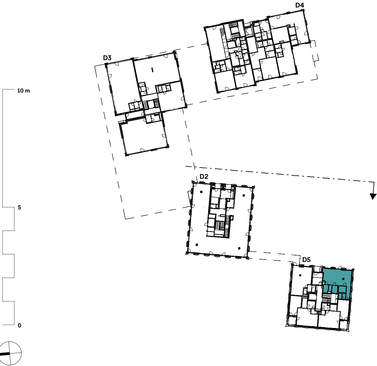
PŮDORYS 1.NP
