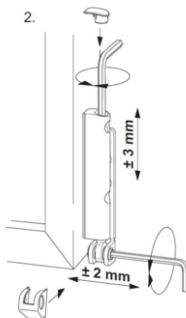
2. Ložisko bez seřizení přítlaku
