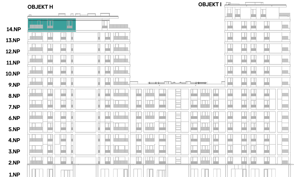
POHLED SEVERNÍ
