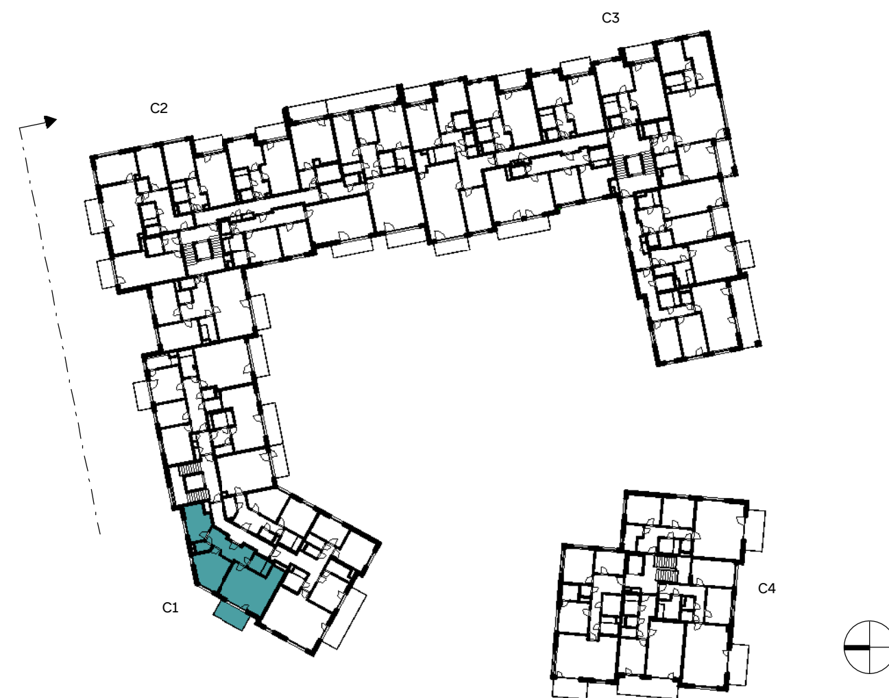
PŮDORYS 2.NP
