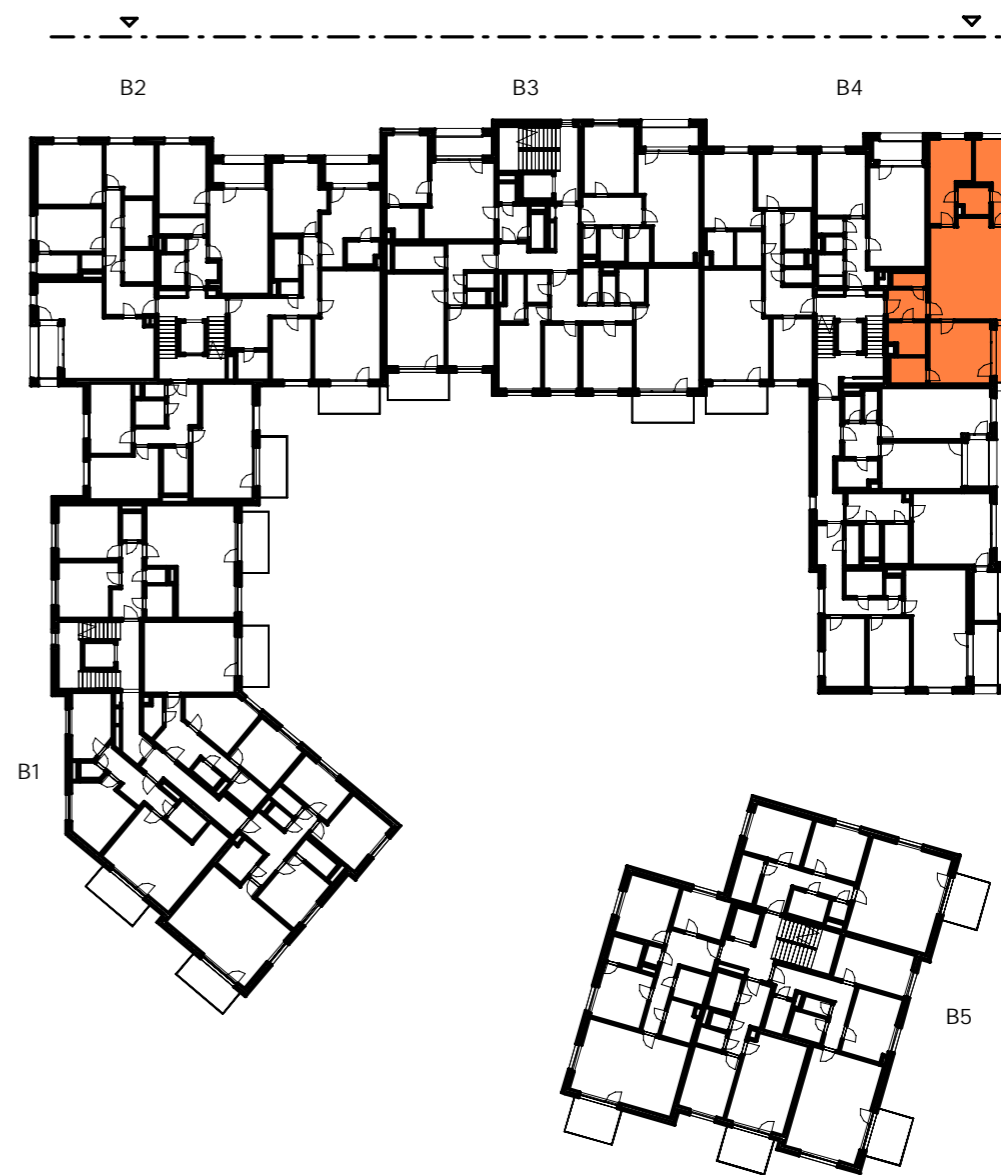
PŮDORYS 2.NP
