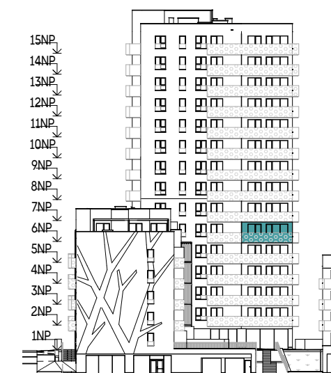
POHLED ZÁPADNÍ
