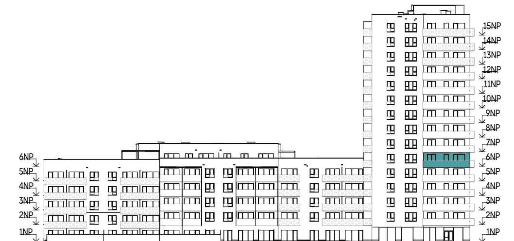
POHLED JIŽNÍ
