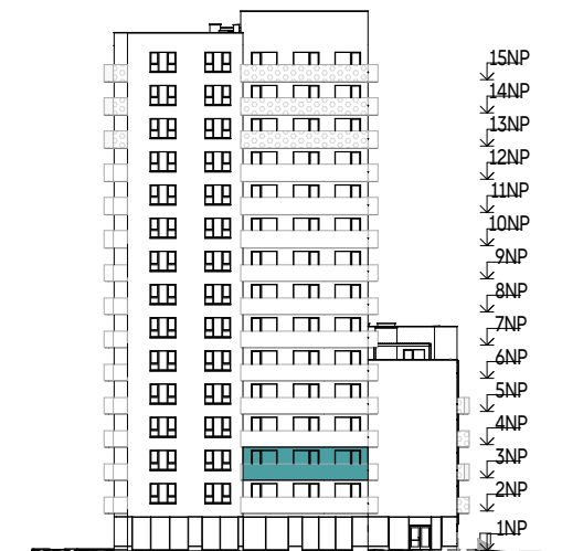
POHLED VÝCHODNÍ
