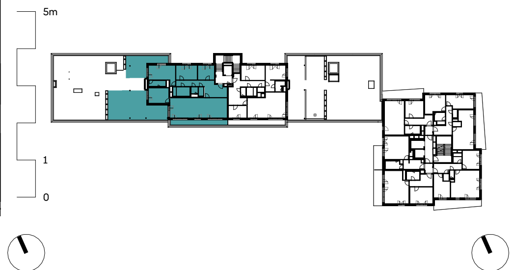
PŮDORYS 6NP
