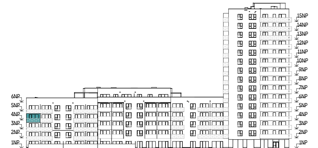
POHLED JIŽNÍ
