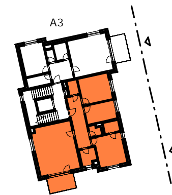
PŮDORYS 2.NP
