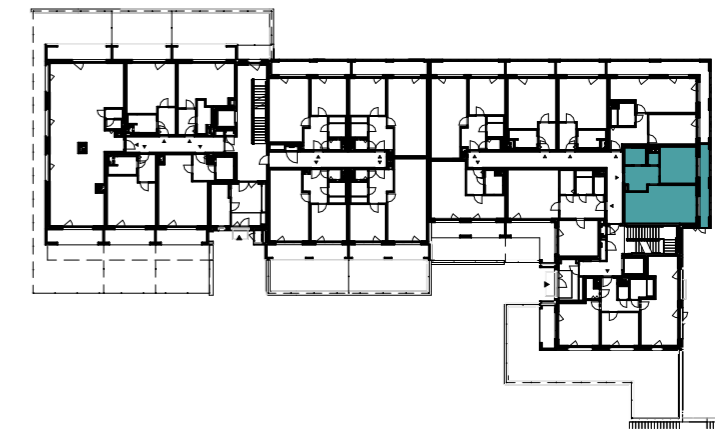
schéma podlaží
